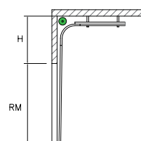
Высокий с верхним расположением вала H = 900 \text{ мм}
