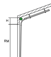
Наклонный H = 490 \text{ мм}
