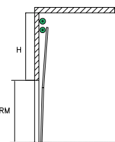
Вертикальный с верхним расположением валов
