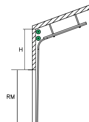
Наклонный высокий с верхним расположением валов H = 1275 \text{ мм}
