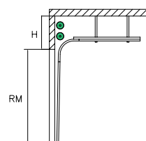
Стандартный H = 840 \text{ мм}
