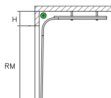
Стандартный H = 410 \text{ мм}
