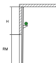
Вертикальный с нижним расположением вала H = RM + 340 \text{ мм}
