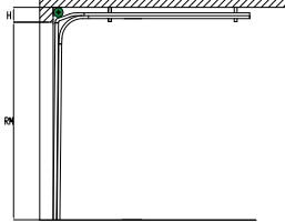
Низкий тип монтажа с передним расположением вала, тип 2
