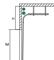
Высокий монтаж с верхним расположением валов H = 1275 \text{ мм}
