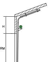
Наклонный высокий с нижним расположением вала
